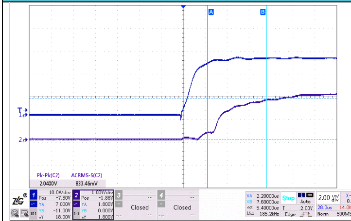
图 3: 响应延迟时间
