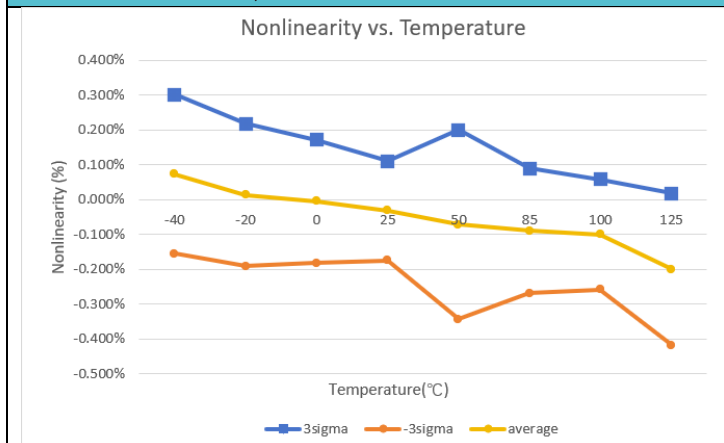
图 3: 非线性 Vs 环境温度
