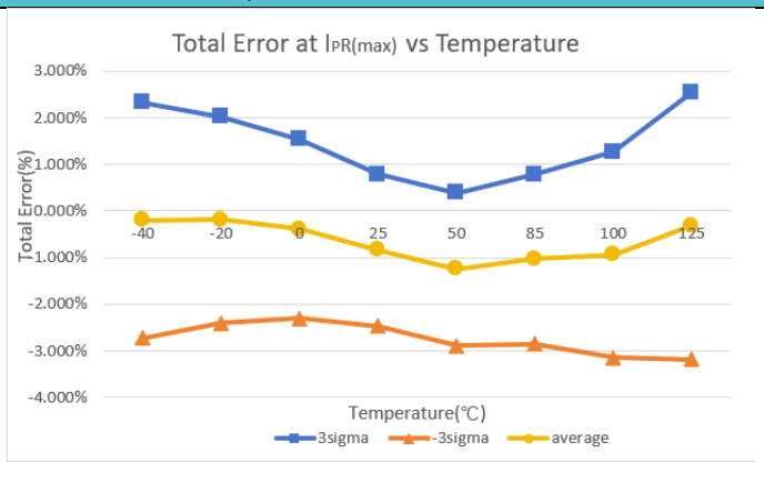
图 4: 总误差 Vs 环境温度
