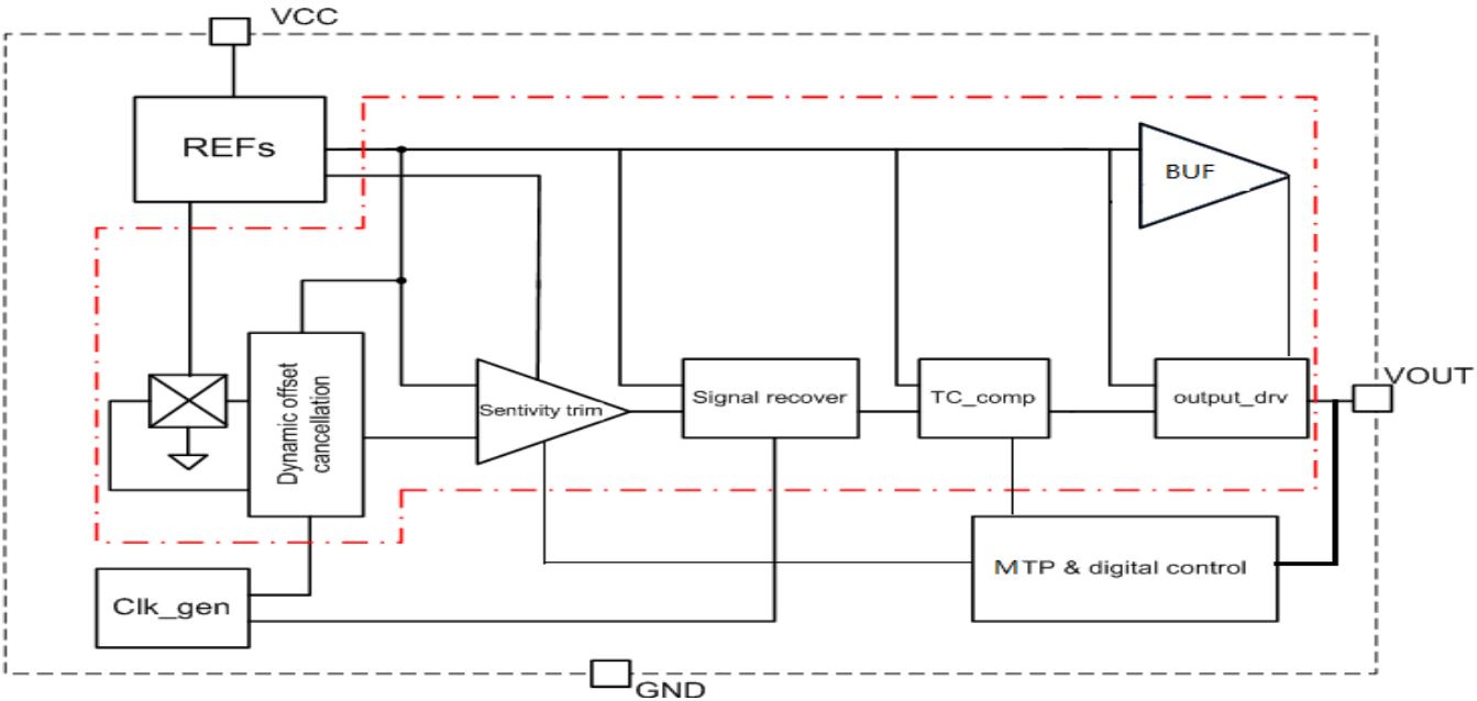
功能框图
