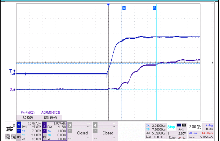
图 4: 上电响应时间
