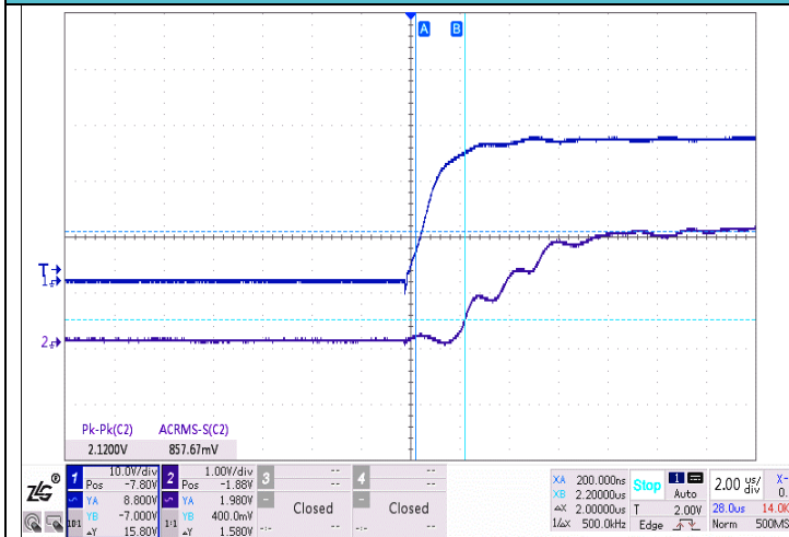
图 3: 响应延迟时间
