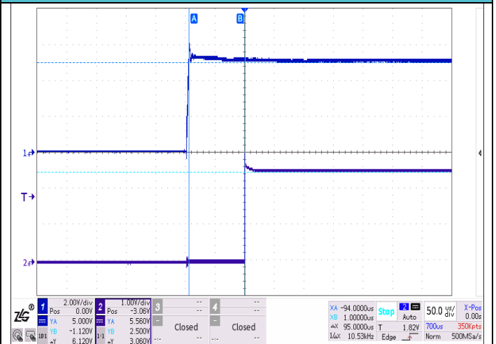
图 4: 上电响应时间
