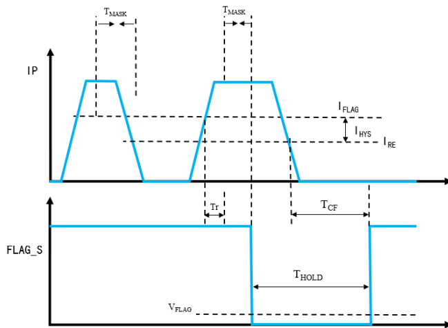
图 3: Tmask 功能启用时 FLAG_S 时序图
